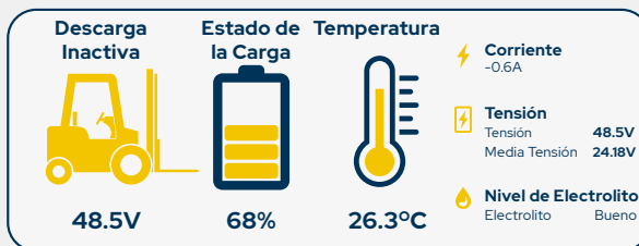
Panel de instrucciones de Sunlight GLocal de los perfiles de batería y de montacargas
