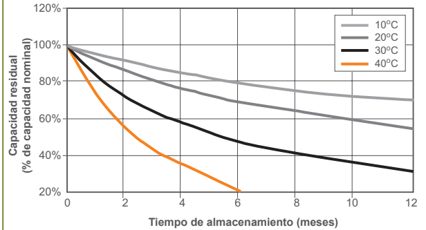
Características de autodescarga
