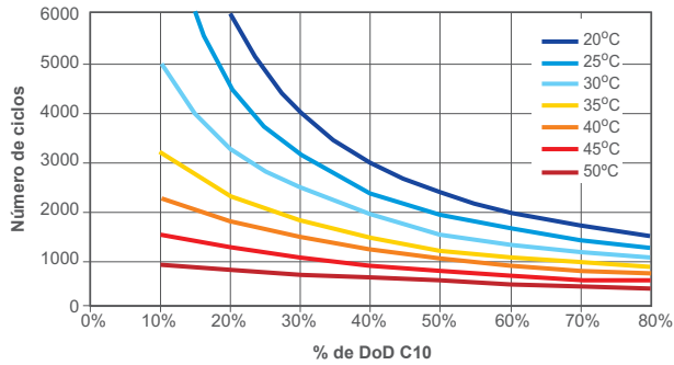
Número de ciclos previstos frente a DoD
