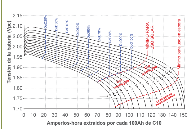
Ajustes de desconexión por baja tensión
