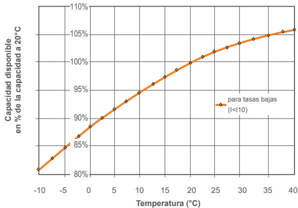
Capacidad frente a temperatura
