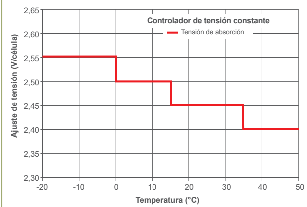
Ajustes de carga para sistemas híbridos
